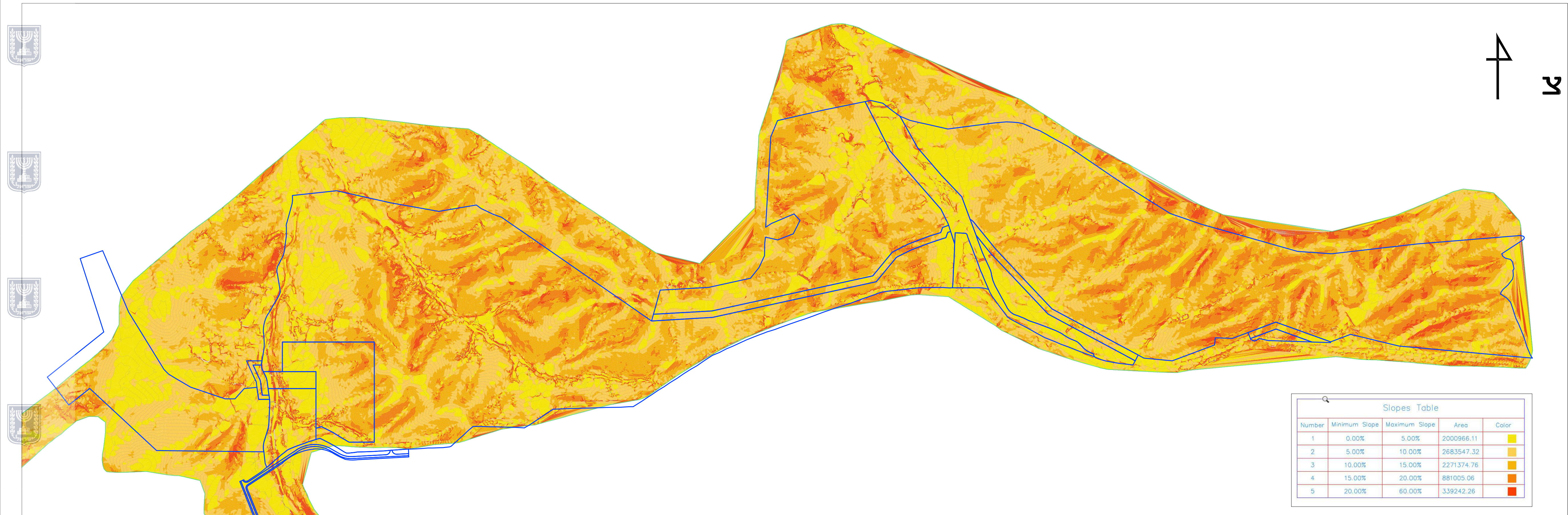
תוכנית שיפועי קרקע 1:10000
