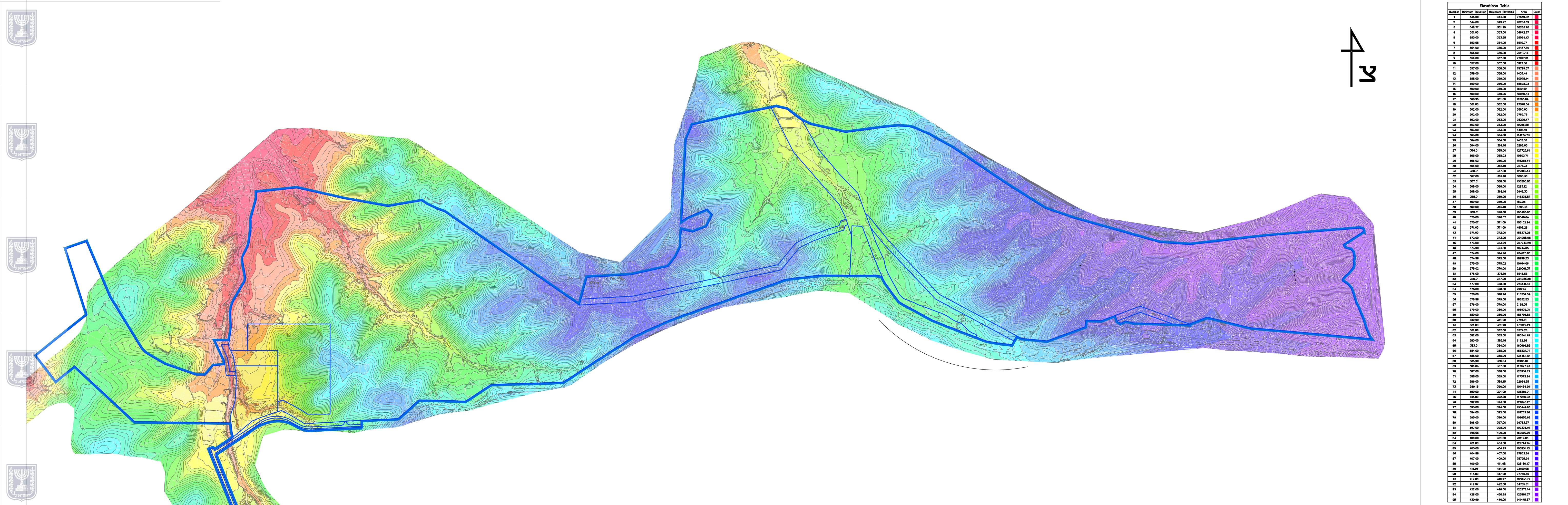
תוכנית רומי קרקע 1:10000
